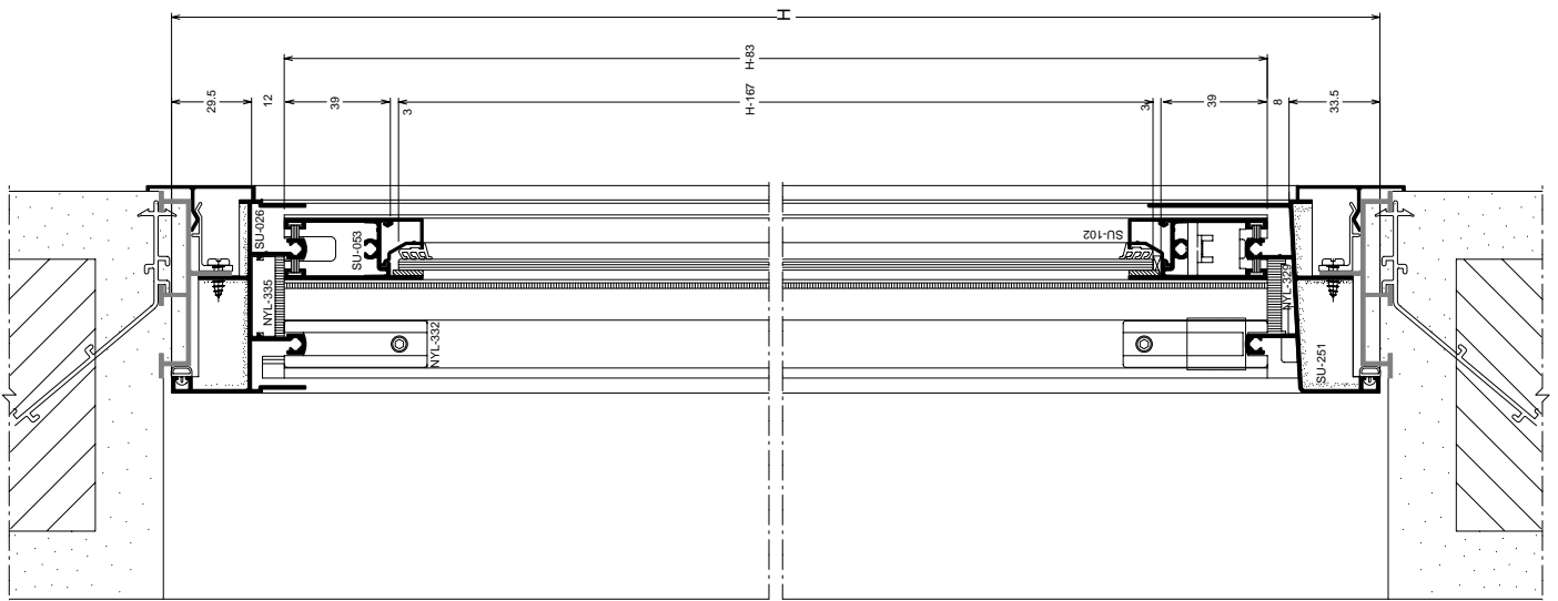
CORTE - 02
