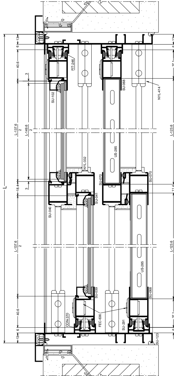
CORTE - 05
