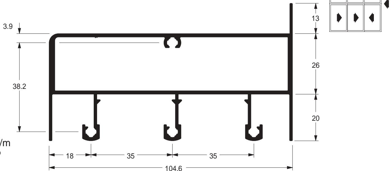
Travessa bandeira / marco / correr 3
