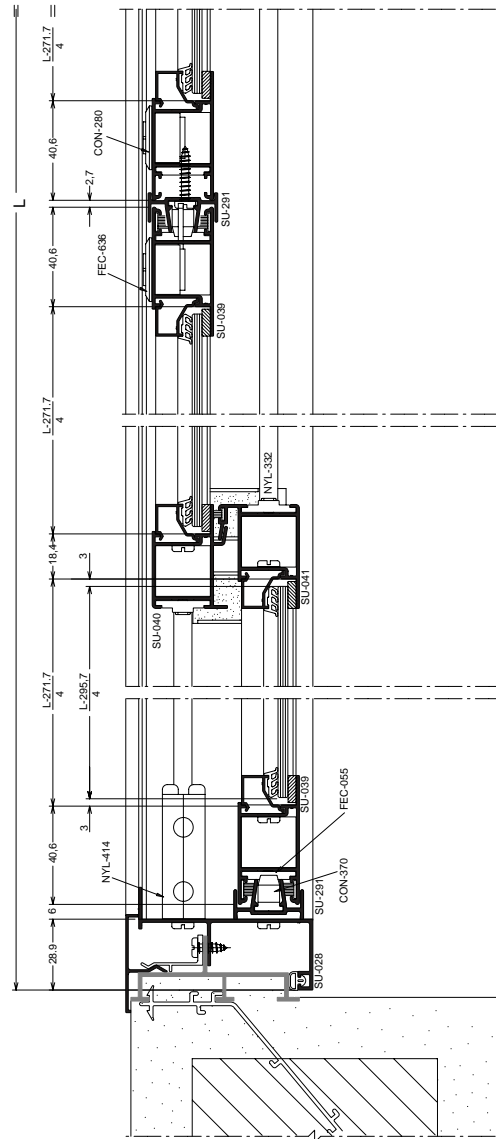
CORTE - 03
